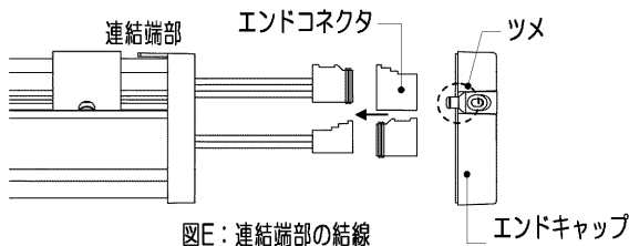
図E：連結端部の結線
