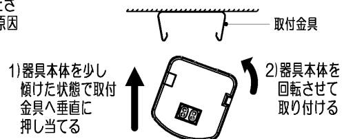
図C：器具本体と取付金具の取り付け
