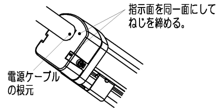
図B：連結端部の結線
