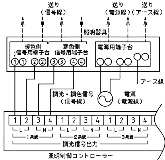
(図15) 照明制御コントローラーとの結線図
