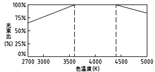
(図16) 調光調色の範囲
