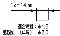
第5図 (単線) φ2.0
