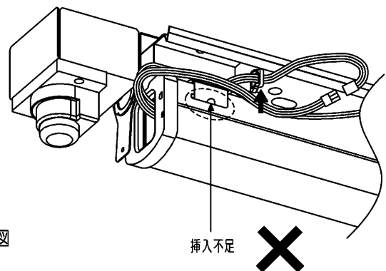
第5図：本体と取付けばねの取り付け
