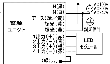
結線図2
