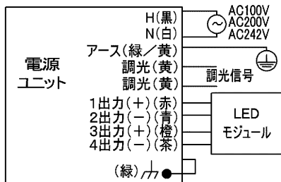
結線図1
