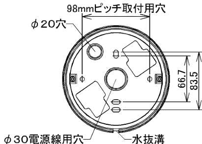
図-2 取付寸法図
