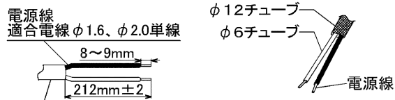
図-3 電源線皮むき寸法 図-4 耐熱保護チューブの取り付け方
