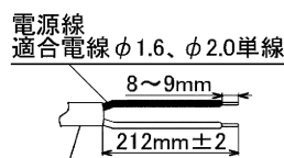
図-3 電源線皮むき寸法
