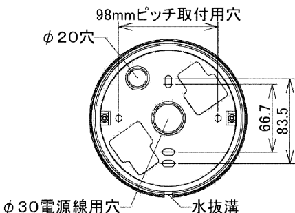
図-2 取付寸法図
