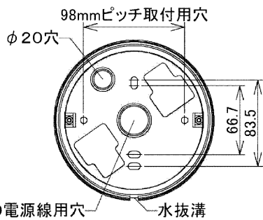
図-2 取付寸法図
