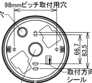
図-3 取付寸法図
