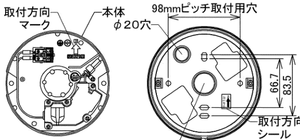
図-2 取付方向
