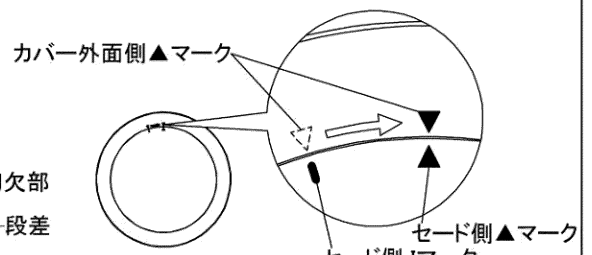
図-7 カバー取り付け固定位置
