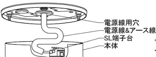
図-5 コード曲げ癖
