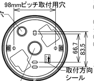
図-3 取付寸法図
