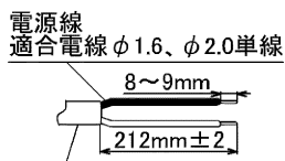
図-4 電源線皮むき寸法
