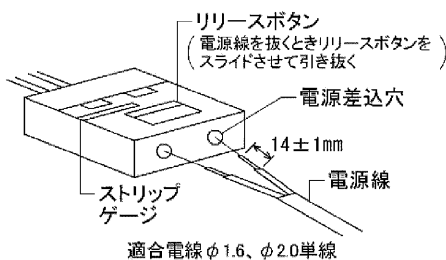
図-4 SL端子台
