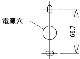
図-2 取付寸法図
