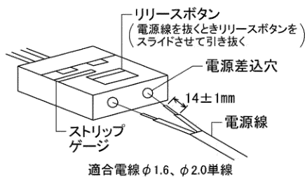
図-4 SL端子台
