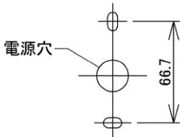
図-2 取付寸法図
