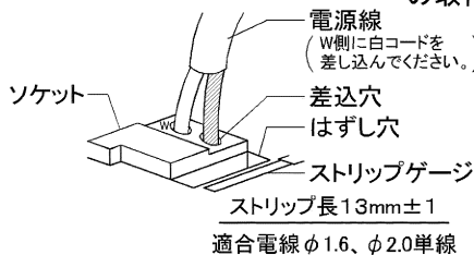
図-6 電源線接続方法
