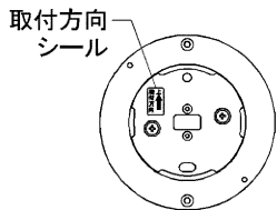
図-2 取付方向
