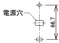
図-3 取付寸法図
