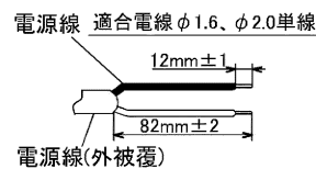
図-4 電源線皮むき寸法
