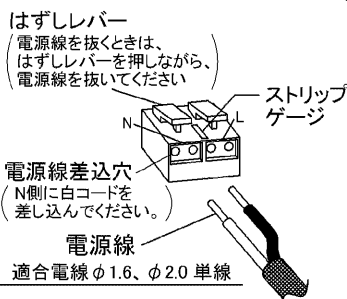
図-5 SL端子台
