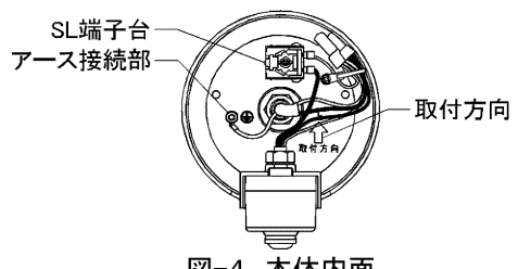
図-4 本体内部
