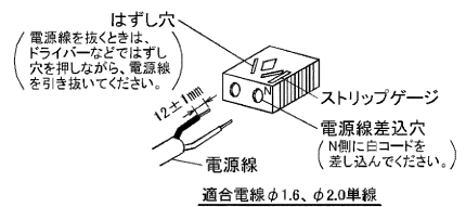
図-3 SL端子台
