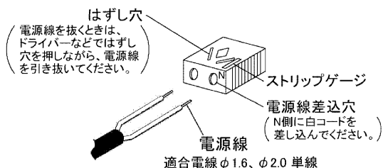
図-5 SL端子台
