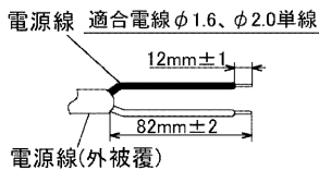
図-3 電源線皮むき寸法
