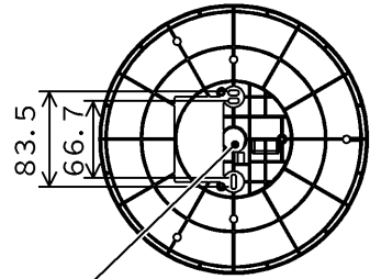
取り付け寸法図
