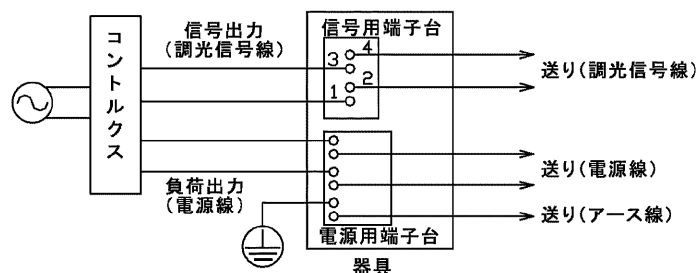
調光制御装置との結線図 (図10)
