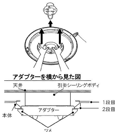
角形・丸形引掛シーリングボディ
