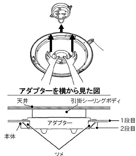
埋込引掛シーリングボディ
