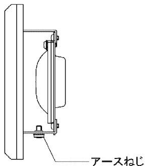
図-3 本体側面
