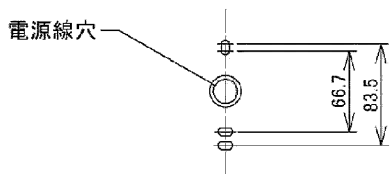
図-3 取り付け寸法図
