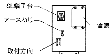
図-7 本体内面
