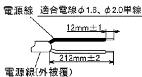
図-4 電源線皮むき寸法
