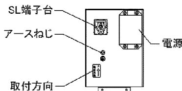
図-7 本体内部
