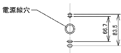
図-3 取り付け寸法図
