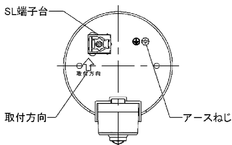
図-3 本体内面
