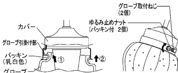
図-5 グローブの取り付け方
