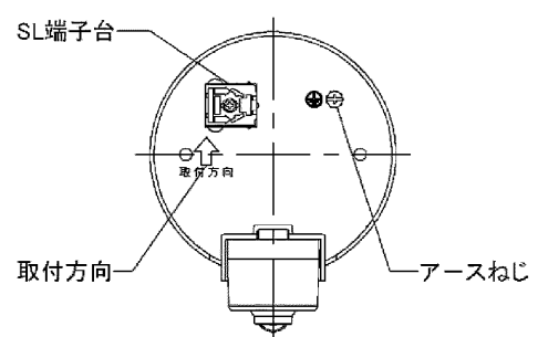
図-3 本体内部
