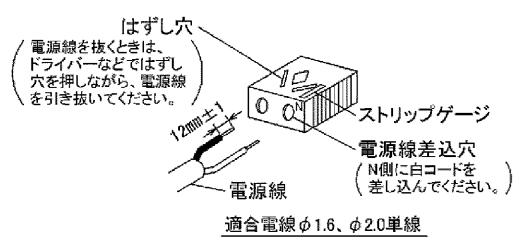
図-4 SL端子台
