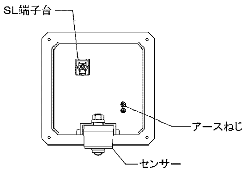
図-2 本体内部
