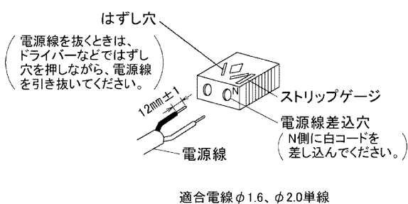
図-4 SL端子台
