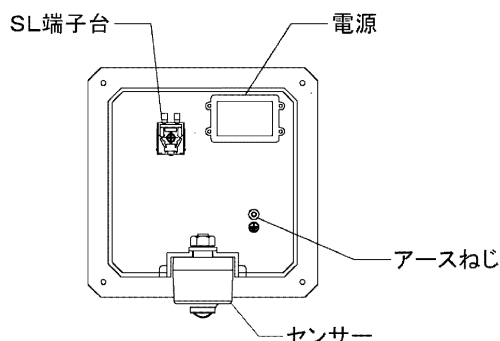
図-2 本体内部
