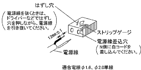
図-4 SL端子台
