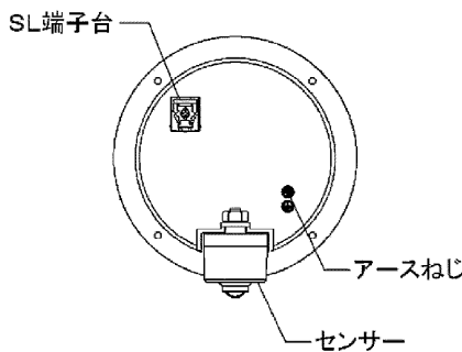
図-2 本体内面
