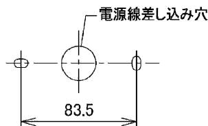
図-3 取り付け寸法図
