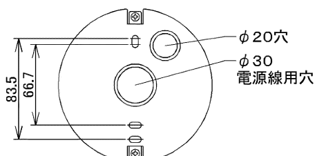
図-3 取付寸法図
