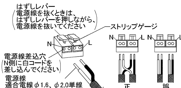
図-4 SL端子台
