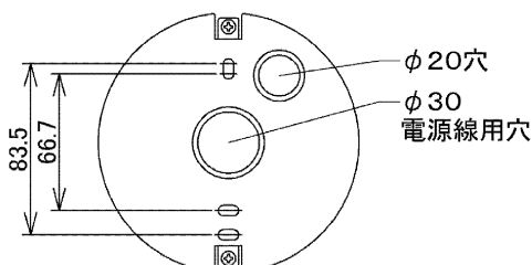
図-3 取付寸法図
