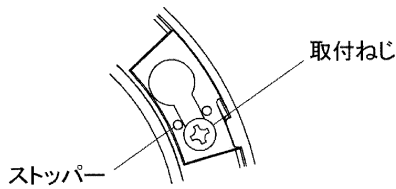
図-7 サポートと本体の取り付けかた
