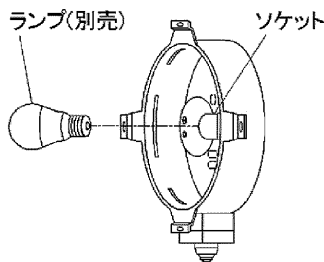
図-5 ランプの取り付け
