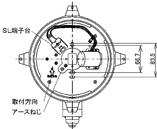
図-2 本体内部
