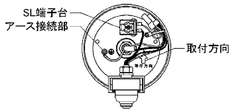
図-4 本体内部
