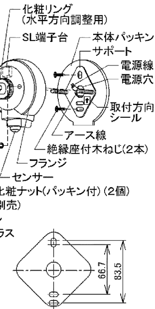
図-2 取り付け寸法図
