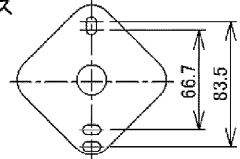
図-2 取り付け寸法図
