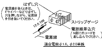
図-3 SL端子台
