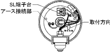
図-4 本体内部
