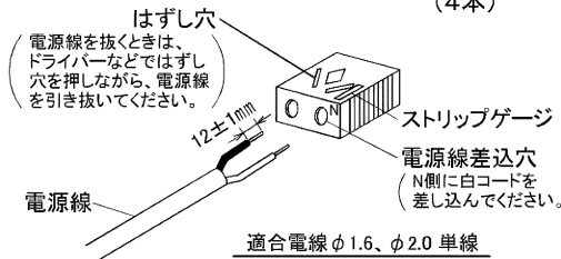
図-2 SL端子台
