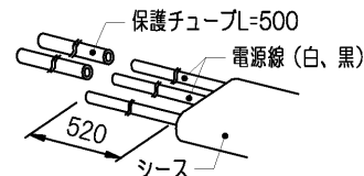
第3図（器具内送りの場合）
