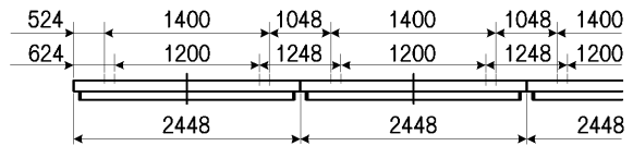
連結寸法図
