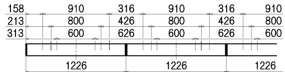
連結寸法図
