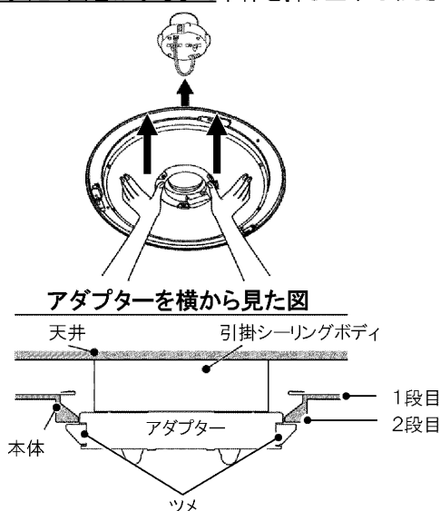
角形・丸形引掛シーリングボディ
