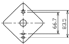
図-2 取り付け寸法図
