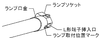
図-3 ランプの取付
