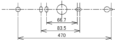
図-5 取り付け寸法図
