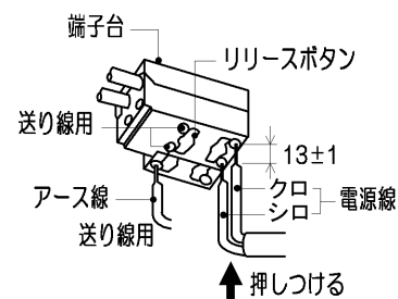
第2図 (適合電線φ1.6, φ2.0 単線)
