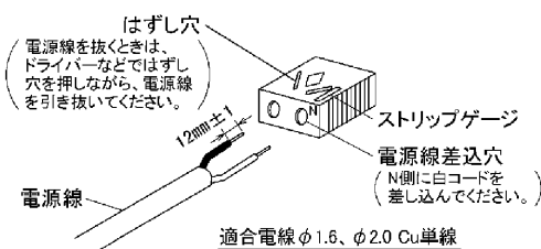
図-3 SL端子台
