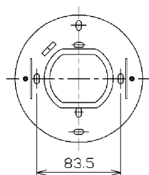
図-2 取り付け寸法図
