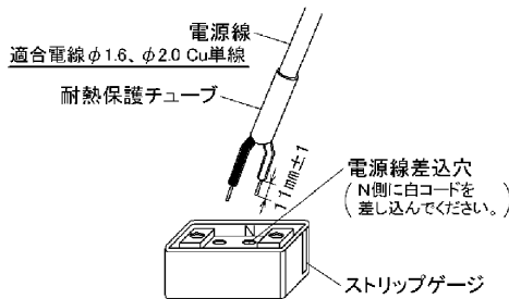
図-2 角形引掛シーリングボディ
