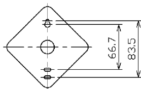
図-2 取り付け寸法図
